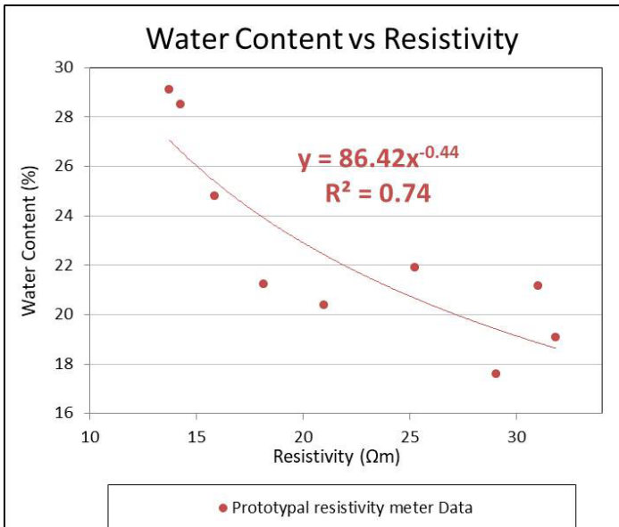
Fig. 2 - Relazione tra contenuto d'acqua e resistività.
